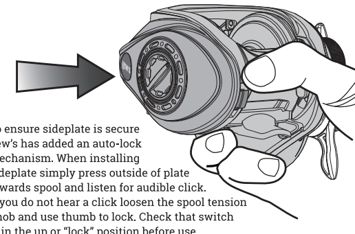
Fig. 2 SLP Sideplate Auto-Lock
